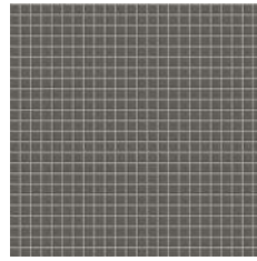
Ematite OPS 2003
