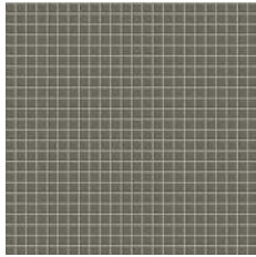
Ramina OPS 2005
