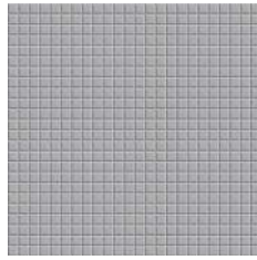
Ankerite OPS 2002
