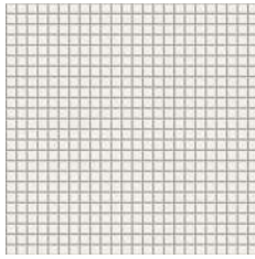
Calcite OPS 2001
