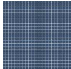
Azzurrite OPS 2012
