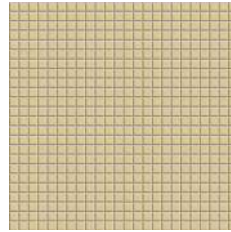
Zirconio OPS 2007
