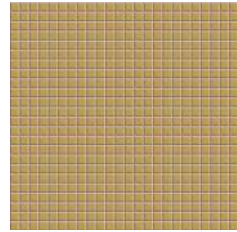
Cerio OPS 2008
