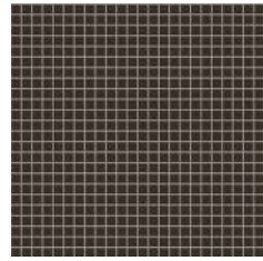
Rutile OPS 2004
